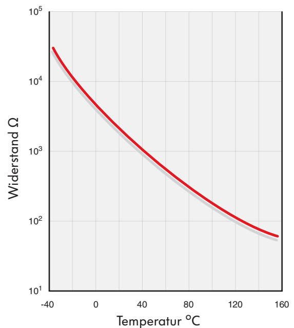
Beispiel einer NTC-Widerstands-Kennlinie
